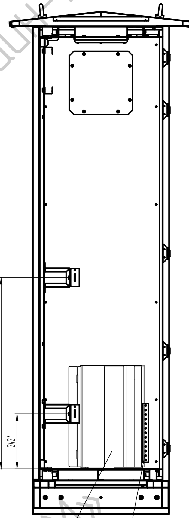
Вид X-X
