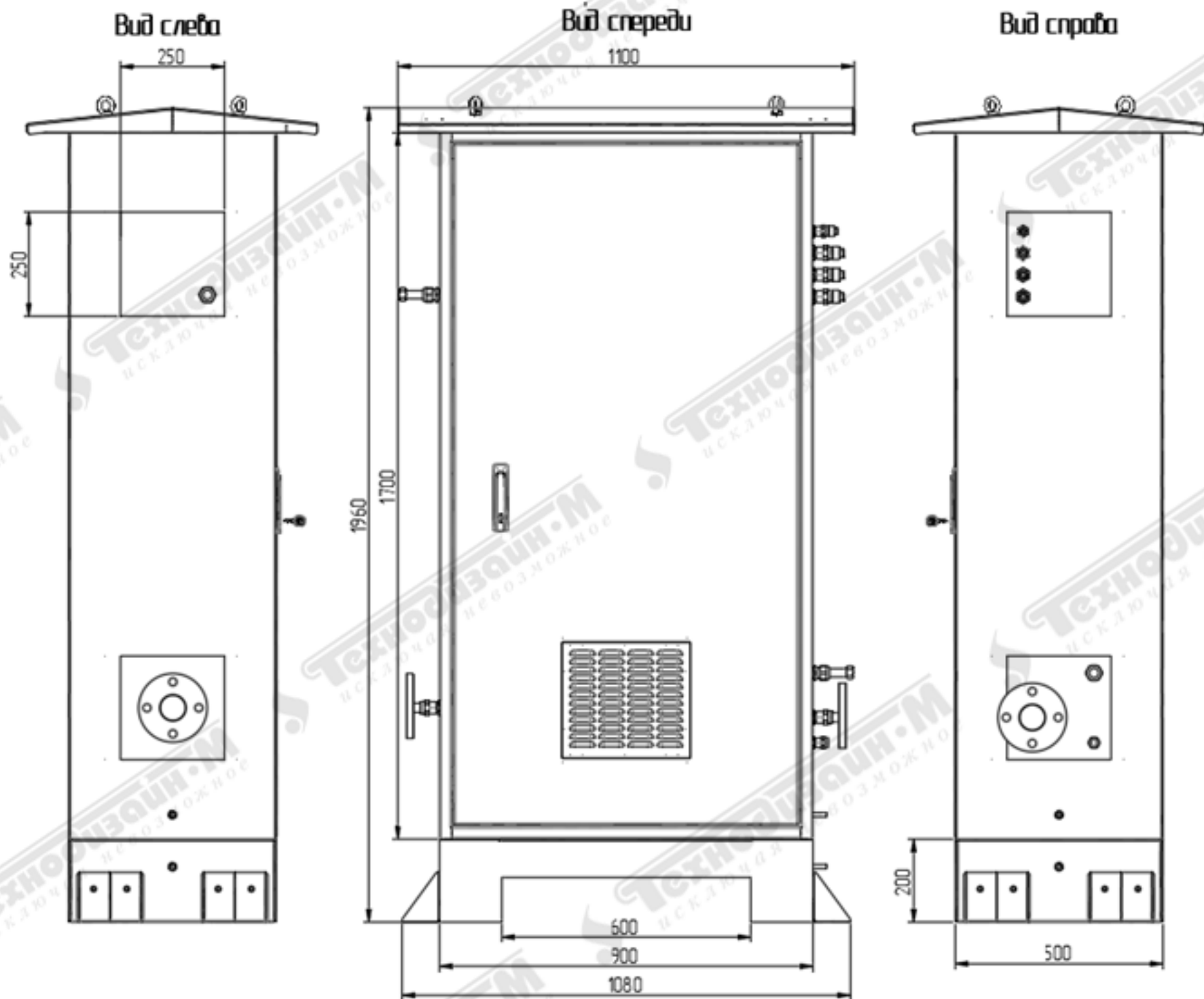
Рисунок 1. Общий вид системы ТДМ-ТШВ-1795-ЕВХ_БМУ-Е+Н.
